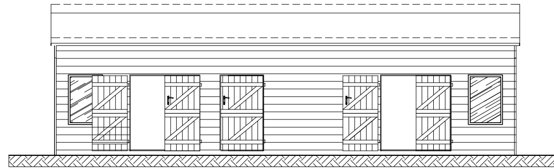
Widok elewacji zachodniej
